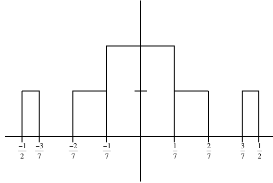
Diagram 1. Journé Dimension Function
